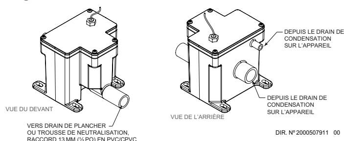
Figure 2-1 Collecteur de condensation
