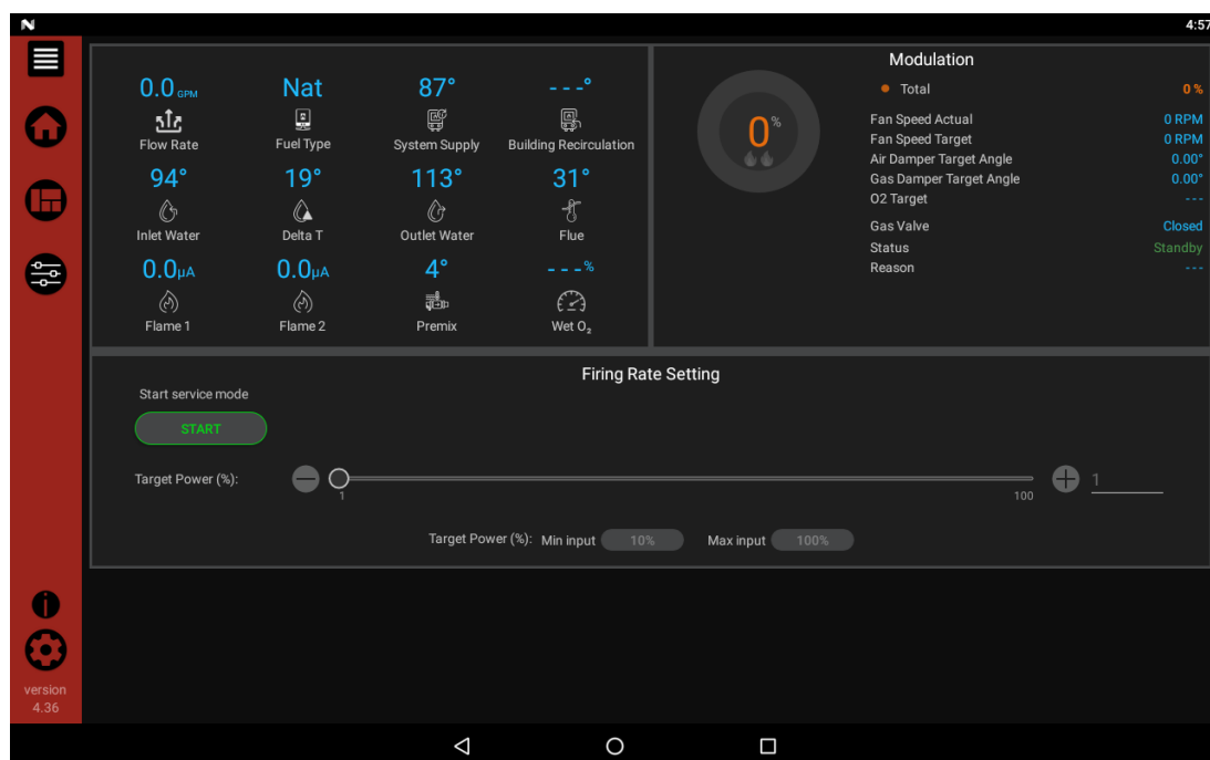
Figure 3-2 Écran d'entretien
