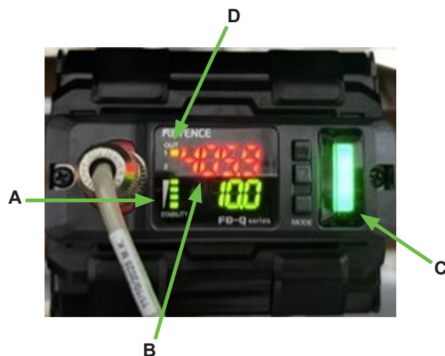
Figure 2-5 AFFICHEUR du capteur de débit ACTIVÉ
