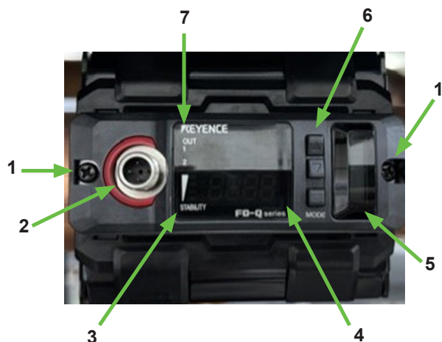
Figure 2-4 AFFICHEUR du capteur de débit DÉSACTIVÉ
