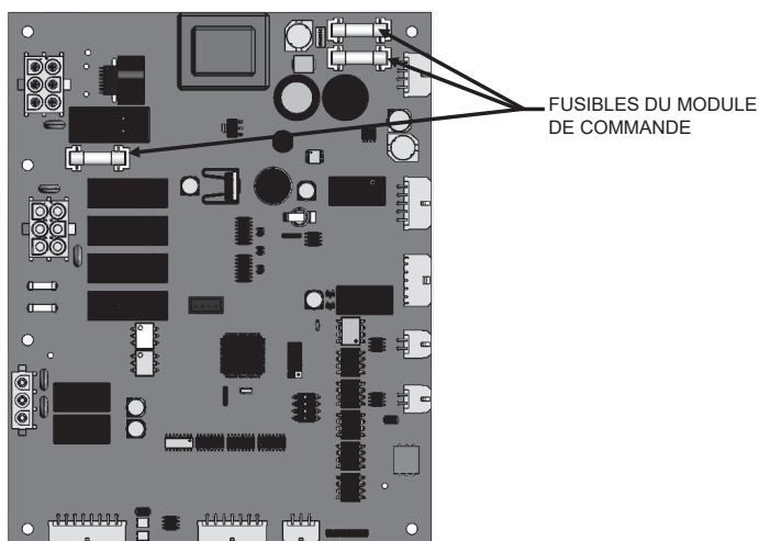
Figure 3-1 Fusibles du module de commande
