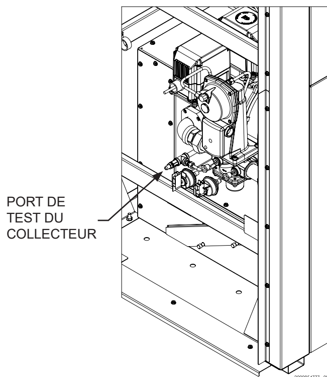
Figure 3-3 Vérification de la pression d'entrée
