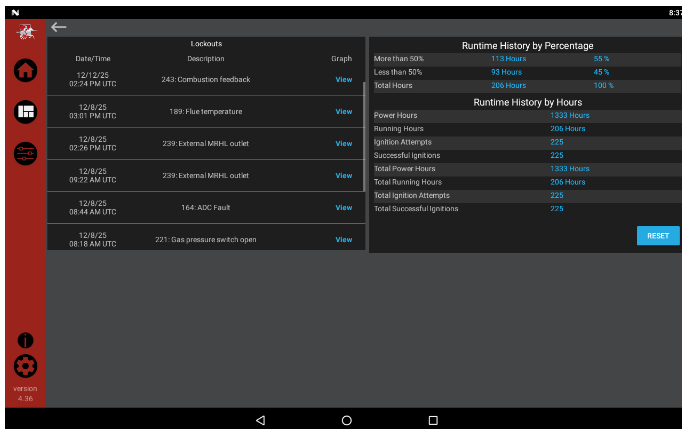
Figure 1-11 Écran History/Runtime History (historique/historique d'exécution)
