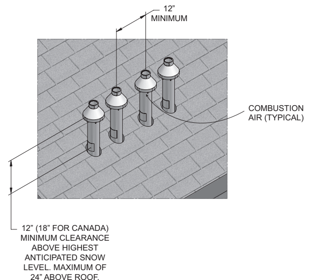
Figure 5-7 Terminaison concentrique, apport d'air et évacuation
