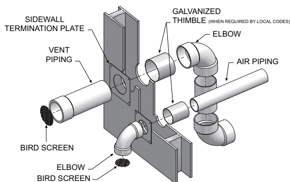
Figure 4-5C Terminaisons murales typiques - PVC/CPVC/ polypropylène ou inox
