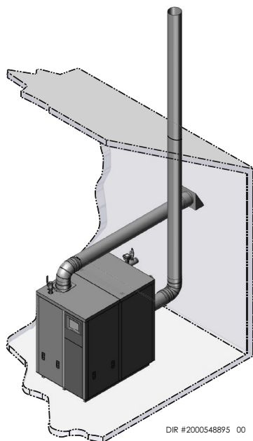
Évent vertical, paroi latérale Air
