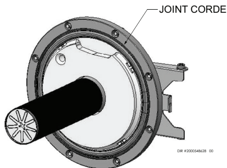
Figure 12-3 Joint en corde - Porte de l'échangeur thermique
