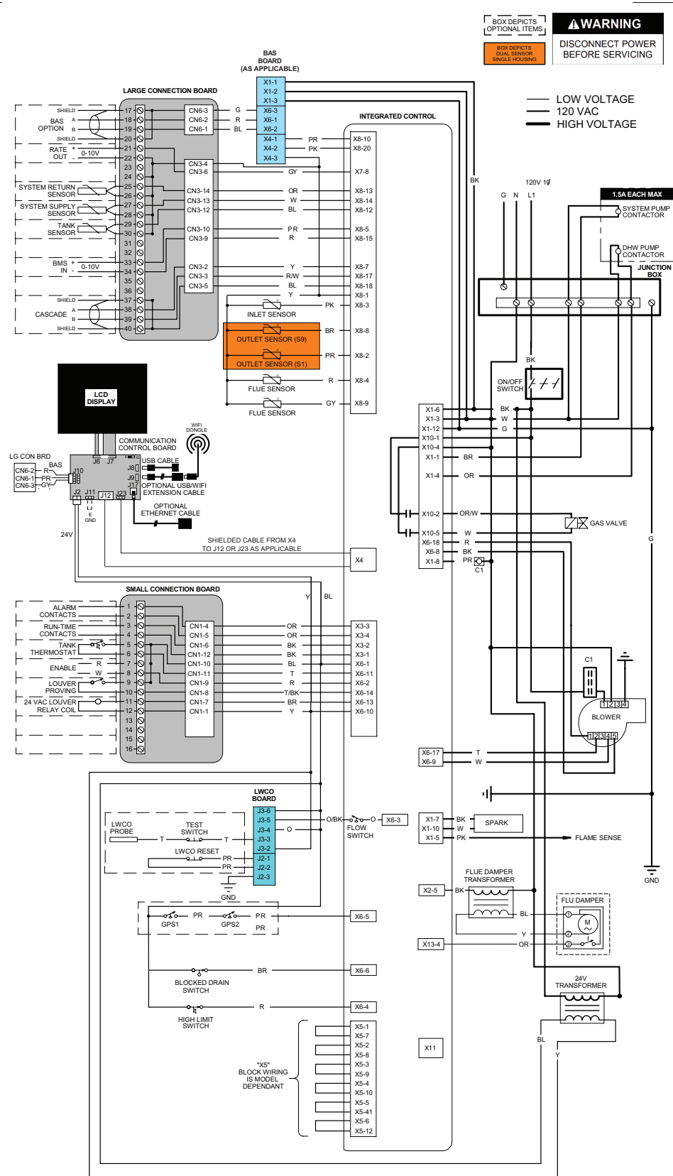
Figure 13-2 Schéma de câblage - 120V - Modèles 1250 et 1500
