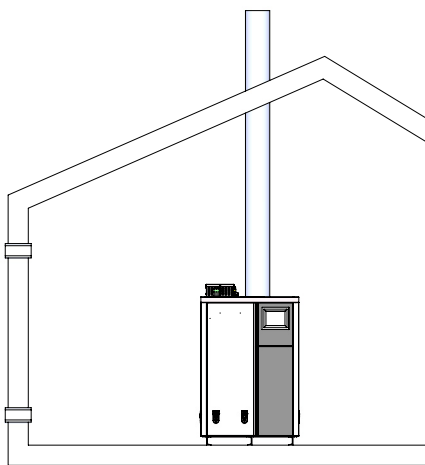
Figure 1-3_Air de combustion tiré directement de l'extérieur
