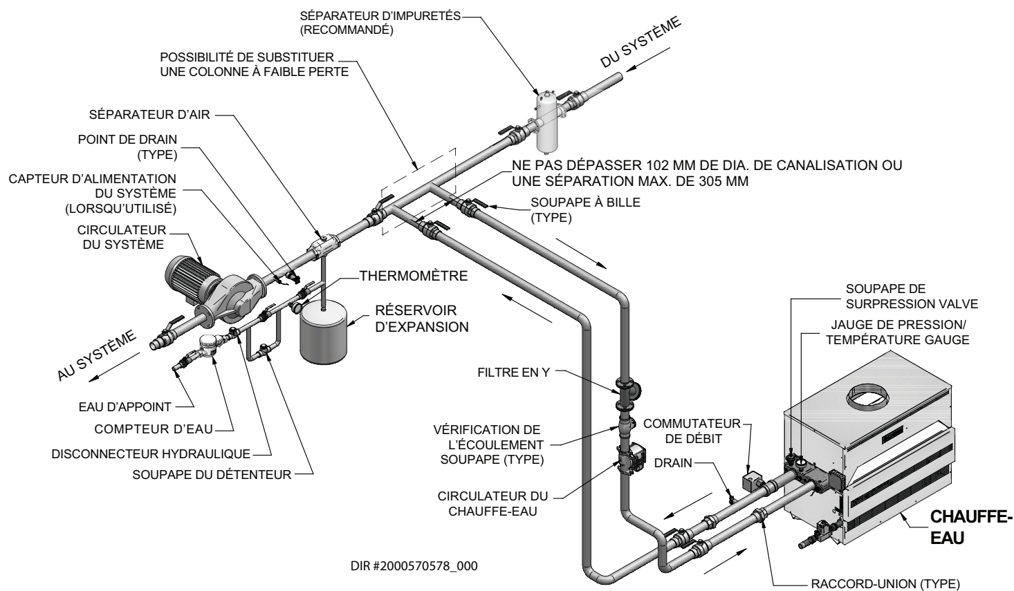
Figure 4-4 Chauffe-eau simple - Canalisations primaires/secondaires
