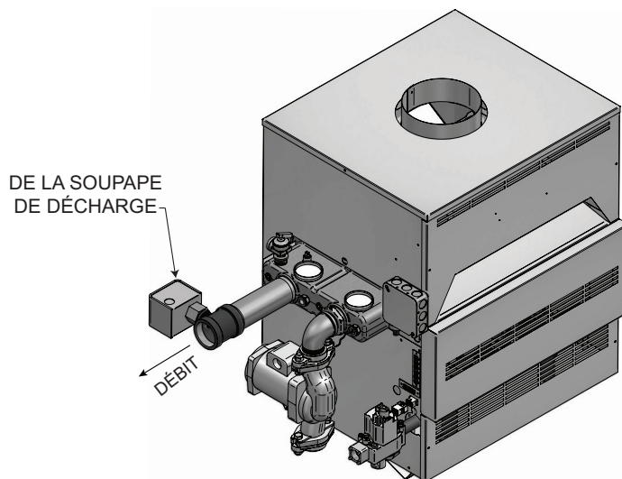
Figure 7-7_Commutateur du débit, chauffe-eau
