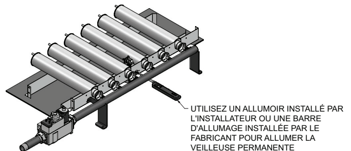
Figure 6-3 Bâton d'allumage
