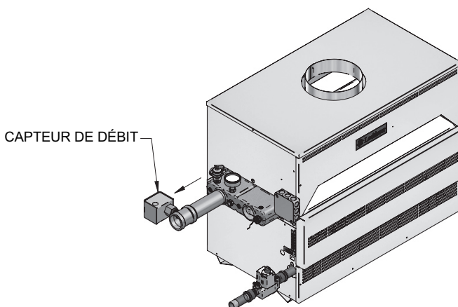
Figure 4-2_Commutateur du débit d'eau - CBN315-500
