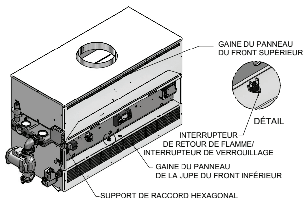
Figure 5-9 Emplacement de l'interrupteur de retour de flamme / de verrouillage de flamme
