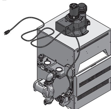
Figure 2-6_CW135 avec ventilation au moyen d'un ventilateur
