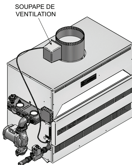
Figure 2-9_CW avec un clapet de ventilation
