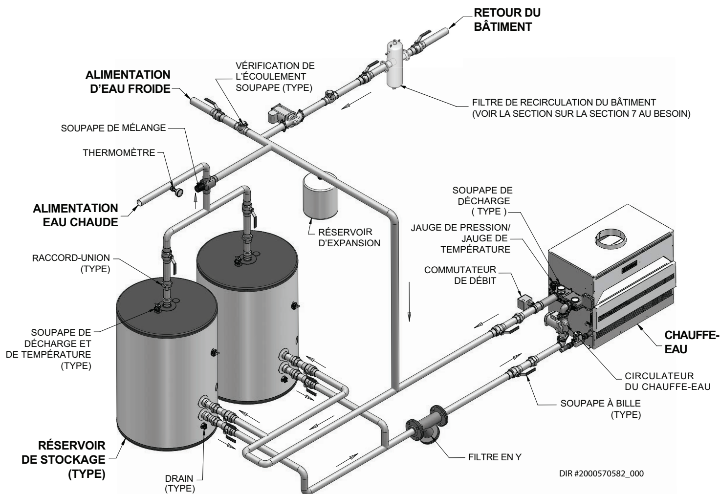
Figure 7-2_Ch chauffe unique_multiple réservoir
