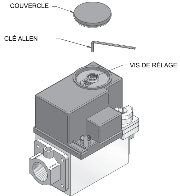
Figure 2-4 Réglage de la vanne du gaz: modèles 400 et 500
