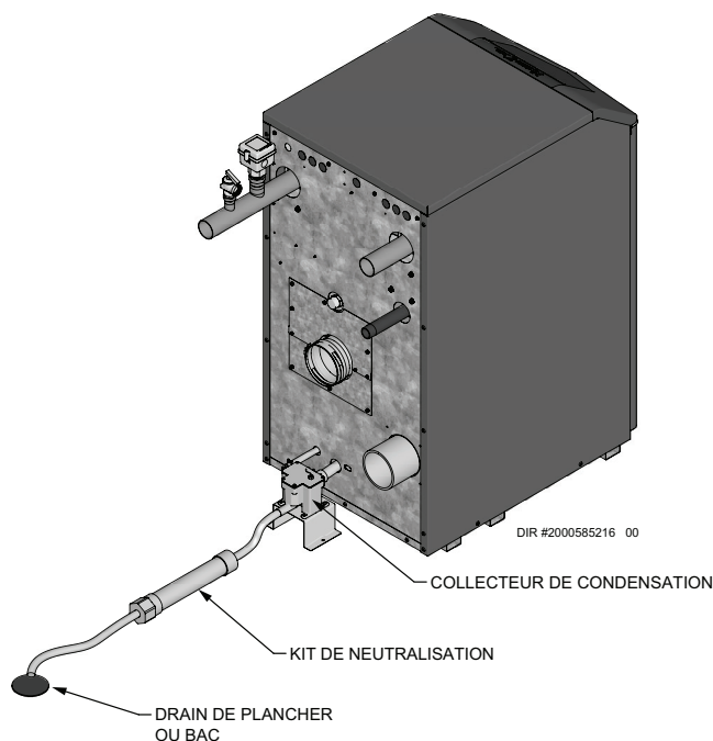
Figure 10-1 Évacuation de la condensation
