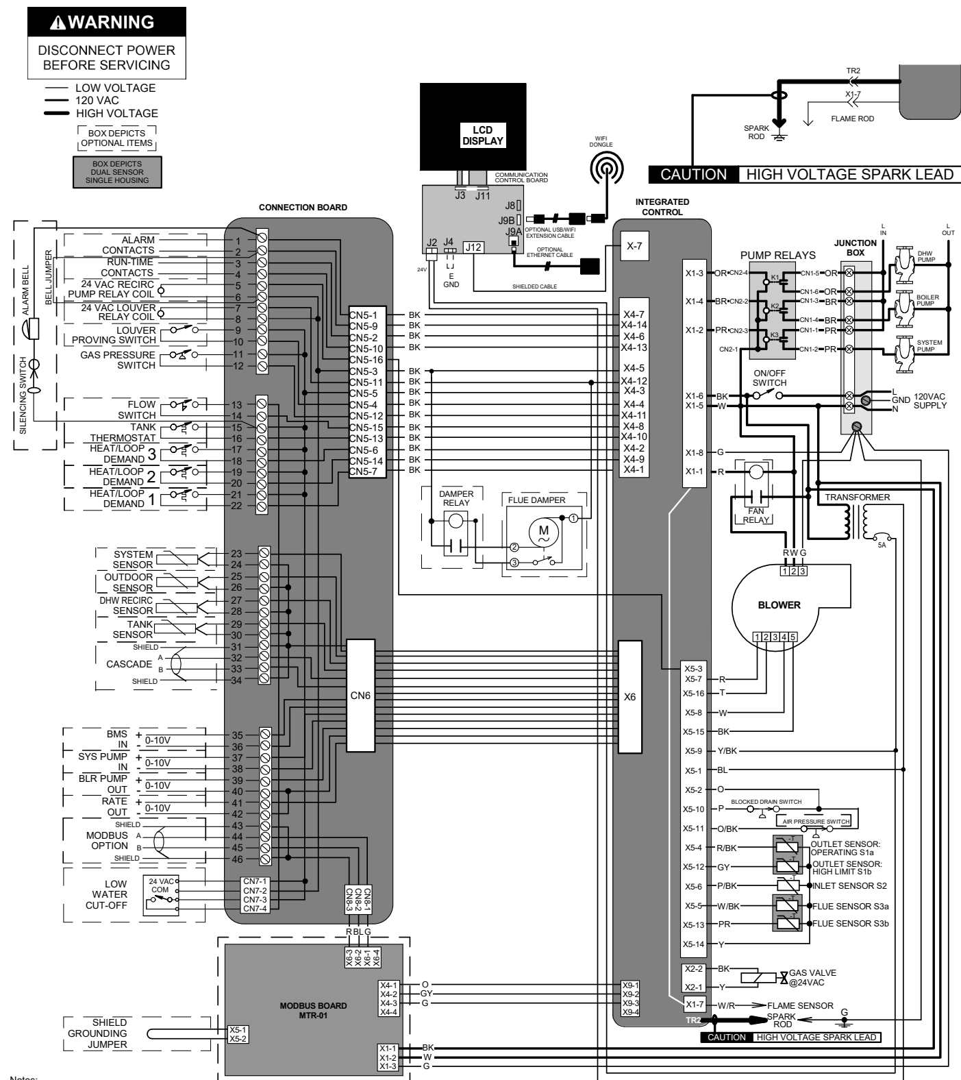
Figure 14-1 Schéma de câblage
