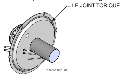
Figure 13-3 Joint torique - Porte de l'échangeur de chaleur
